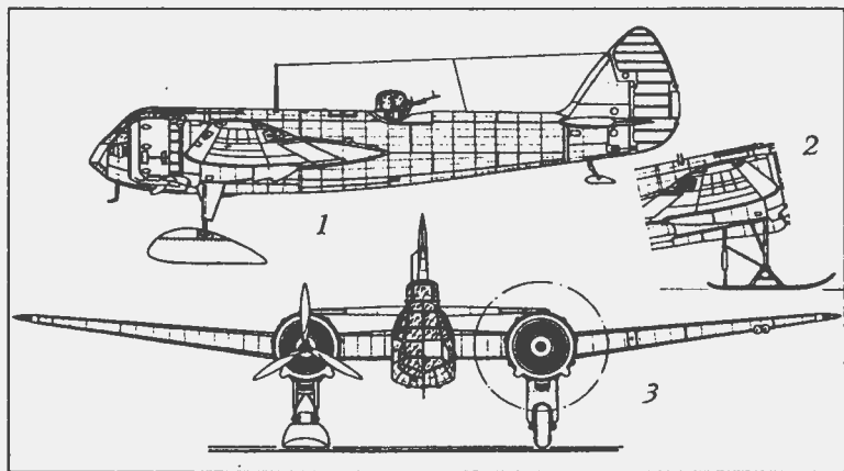
Финский «Бленхейм» Mk.I:
