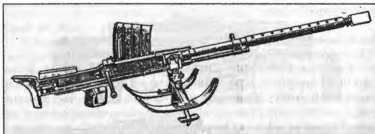
Финское 20-мм противотанковое ружье VKT обр. 1939 г.
