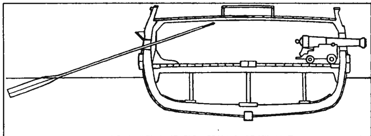
Поперечный разрез прамы «Элефант» (1703 г.)
