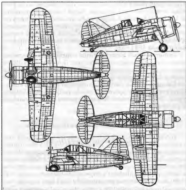
Истребитель В-239 Брюстер «Буффало»
