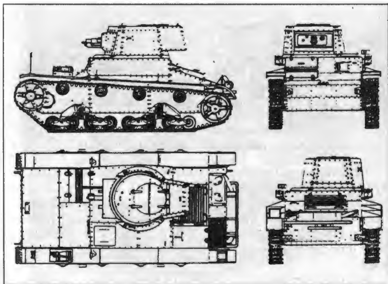
6-тонный «Виккерс», модель E, более поздняя версия B
