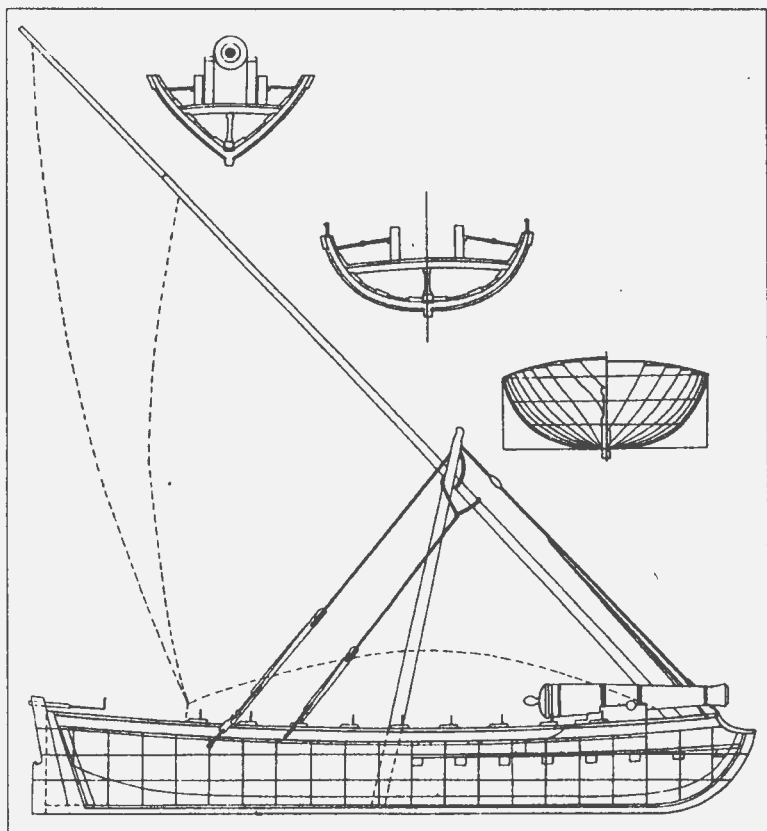
Русская гребная канонерская лодка «малого типа», вооруженная 16-фунтовой пушкой
