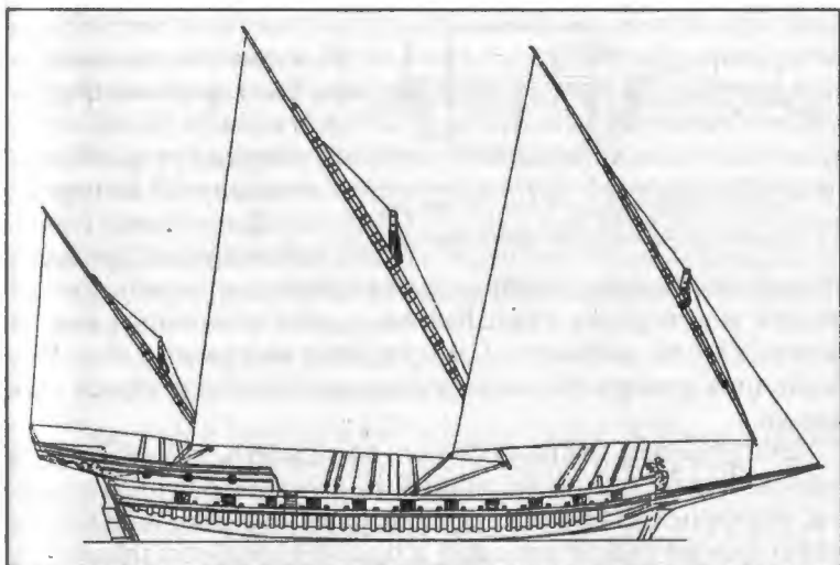
Русская шебека «большого типа»
