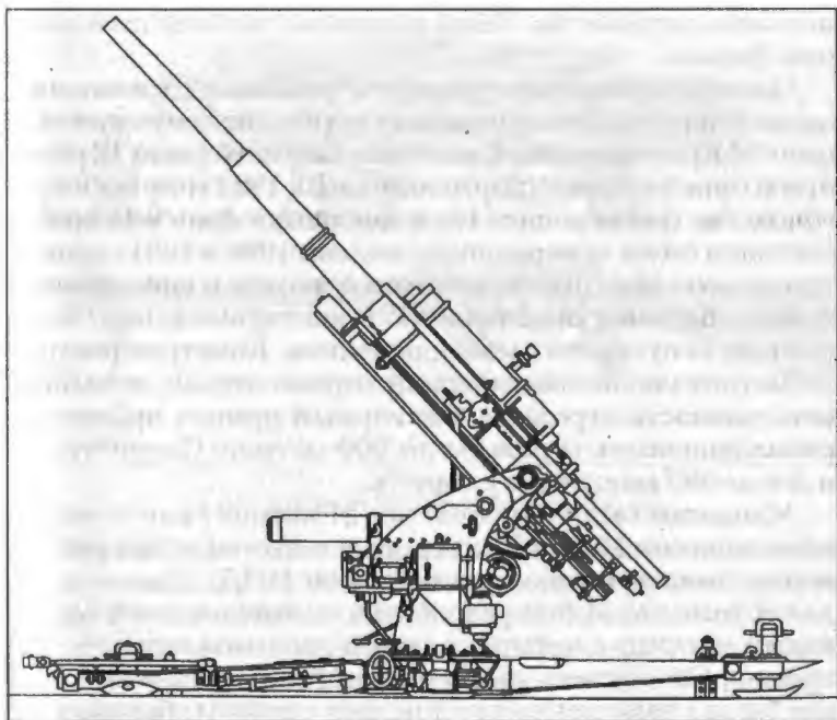
88-мм германская пушка Flak 37 использовалась финнами
