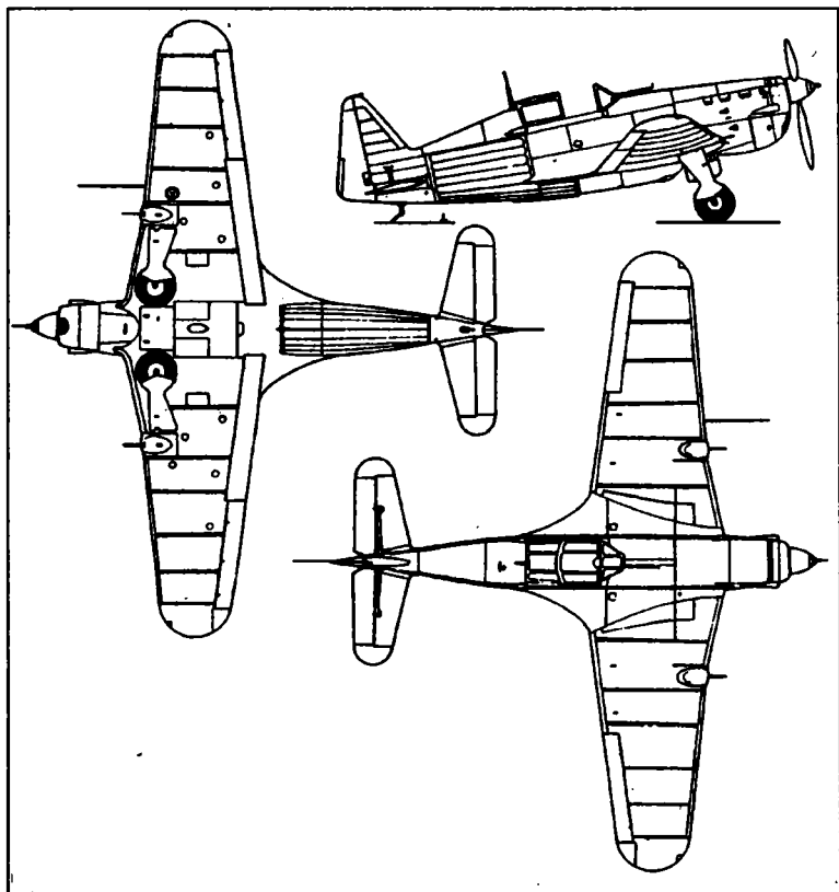
Французский истребитель «Моран» MS-406C1
