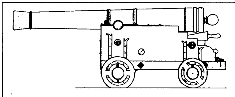
6-фунтовая шведская крепостная пушка
