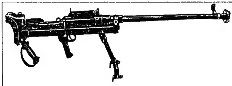
Противотанковое ружье Бойса калибра «.550» (13,37-мм)
