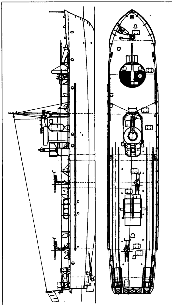
Бронированный морской охотник, специально спроектированный для действий в финских шхерах
