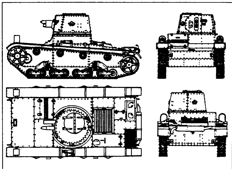
6-тонный «Виккерс», модель E, версия B
