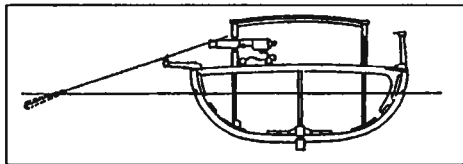
Разрез секретных судов «Охранительный» и «Наступательный»
