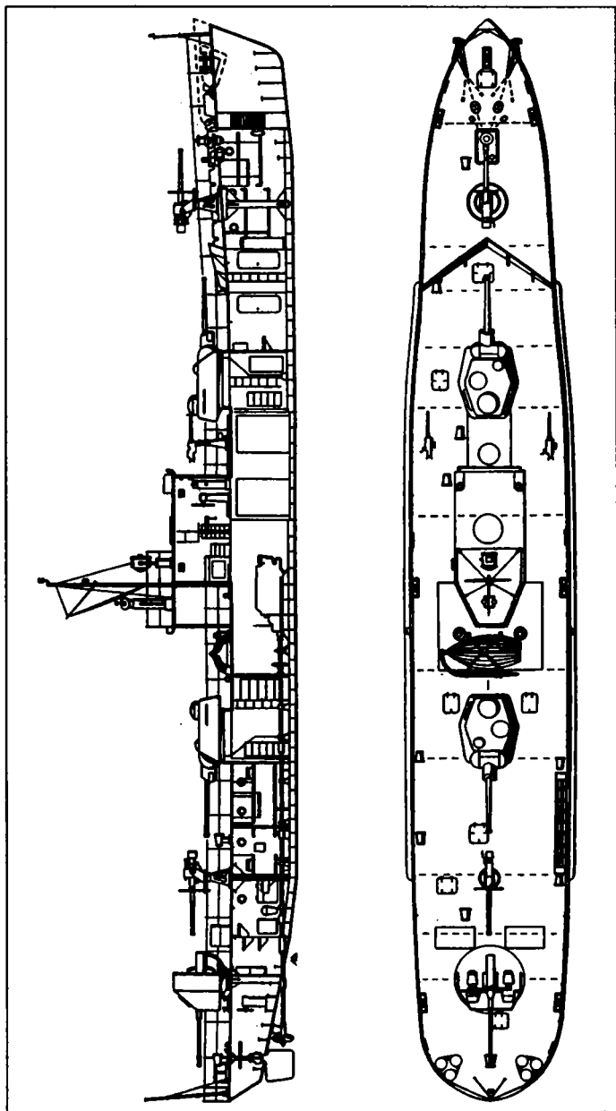
Советская малая канонерская лодка («шхерный монитор»)
