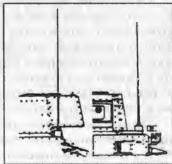
6-тонный «Виккерс», модель E, более поздняя версия B, оборудованный рацмей
