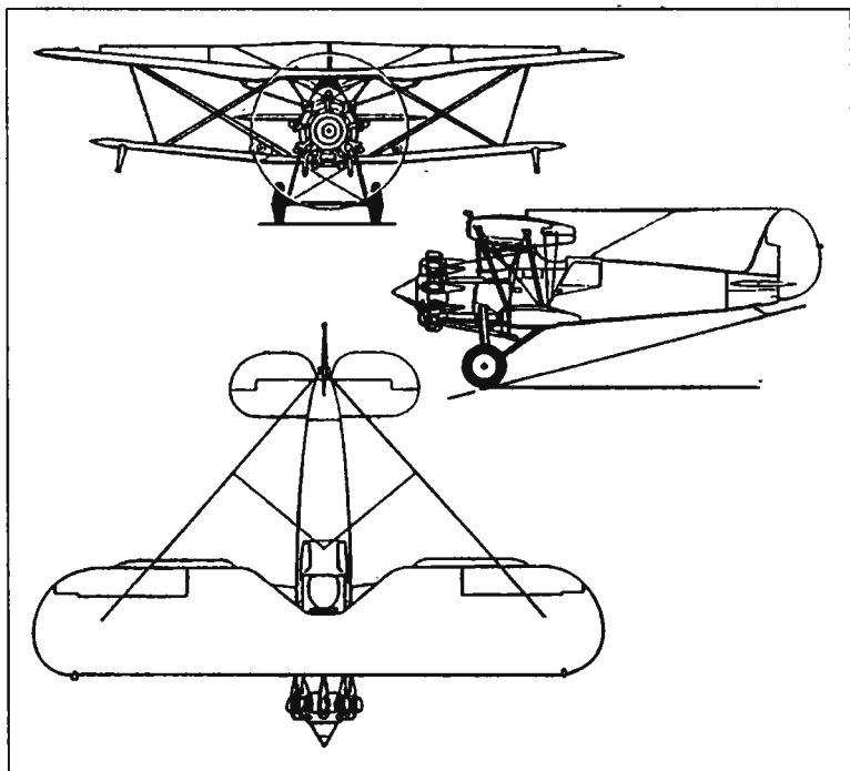
Истребитель Бристоль «Бульдог»
